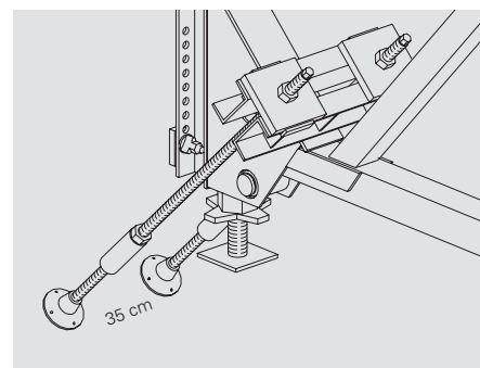
Esempio: Sistema di ancoraggio DW 20 Forza di trazione adm. secondo DIN 18216 2 \times 150 \text{ kN} = 300 \text{ kN} .
