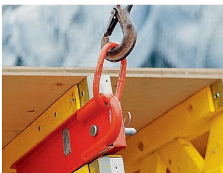
Staffa di sollevamento 24 Portata massima 700 kg, con un angolo di inclinazione delle funi della braca rispetto alla verticale di max. 15°.
