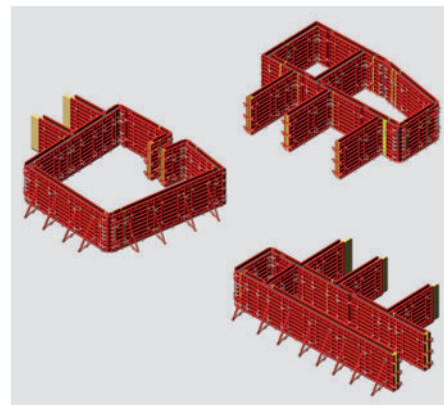
Progettazione tridimensionale con ELPOS e PERI-CAD
