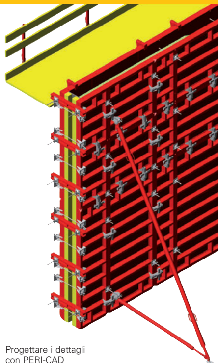
Progettazione tridimensionale con ELPOS e PERI-CAD
