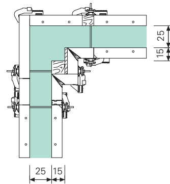
Pilastro incorporato nell'angolo di una parete
