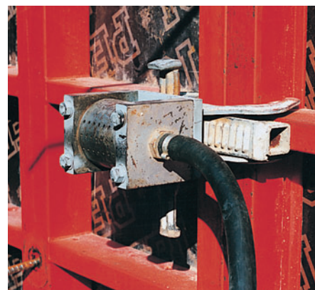
Congiunta ad un vibratore esterno.
